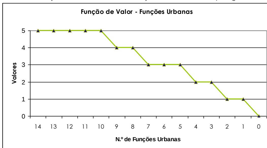
Gráfico 7: Função de Valor do número de funções urbanas existentes por aglomerado
