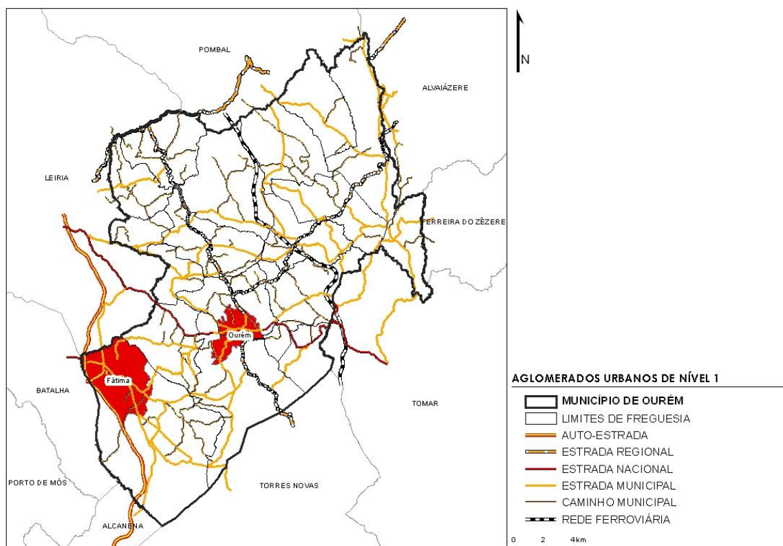
Figura 44: Aglomerados urbanos de nível 1
